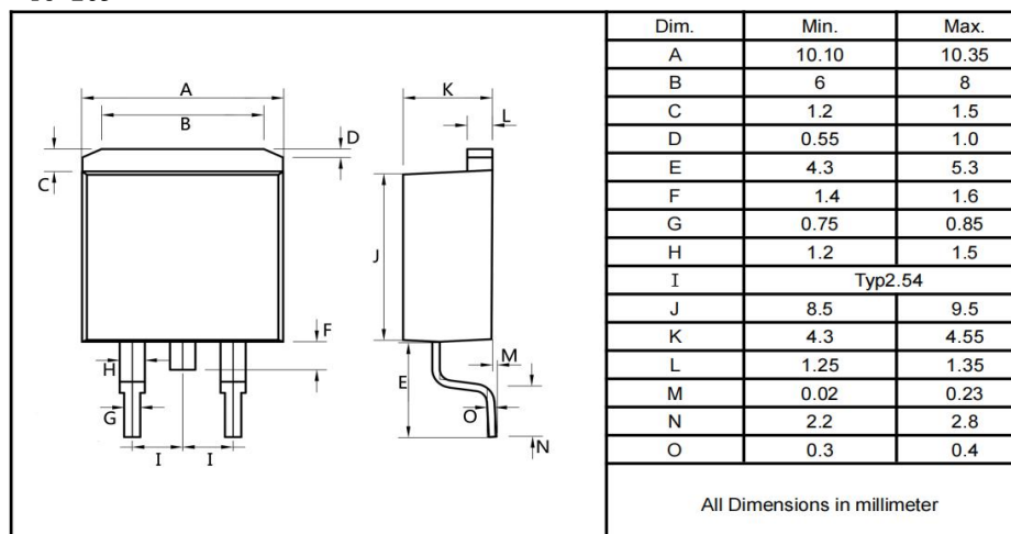
TO-263
